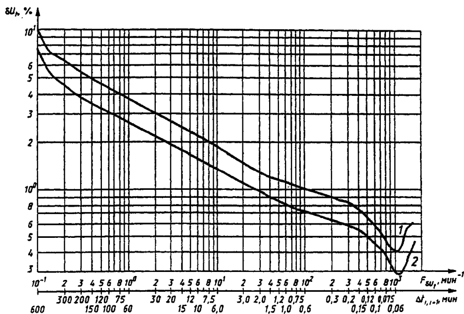
Рисунок 1. Предельно допускаемые размахи изменения напряжения в зависимости от
