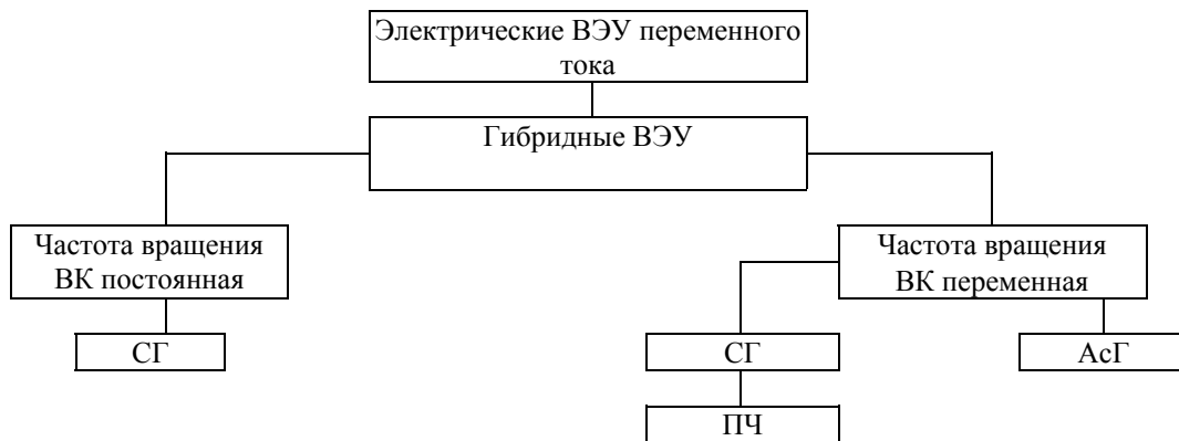
Рисунок 2 — Структурная схема автономных ВЭУ
